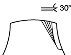
Рис. 22 Заточка ножа
